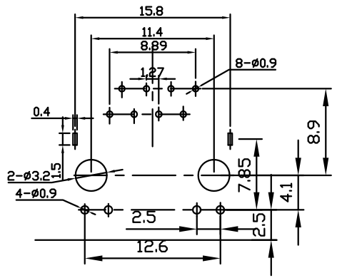
P.C.B参考图 (建议板后1.6mm)
