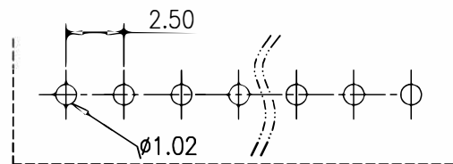
P.C.Board Layout
