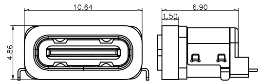
加防水圈示意图
